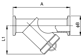
卡箍 Y 型过滤器 Clamped Y-type strainer
